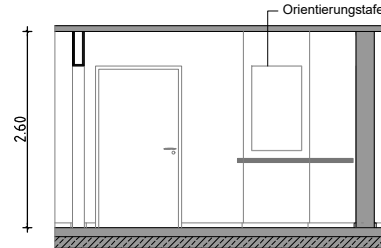
SCHNITT 4-4 Fluchttür der Kurzzeitpflege (abgeschl.)
