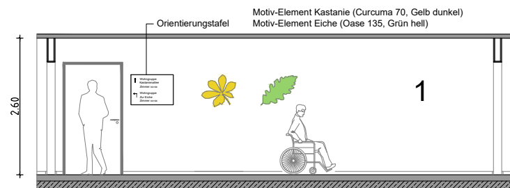
SCHNITT 1-1 Durchgang zu Wohngruppe 2 + 1 Aufzugsfoyer 1.OG
