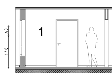
SCHNITT 3-3 Tür zum Pflegebad
