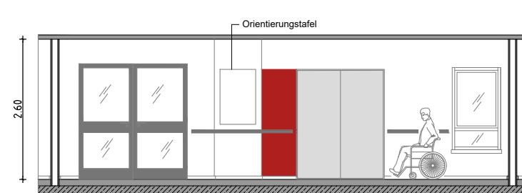
SCHNITT 2-2 Durchgang zum TRH Aufzug
